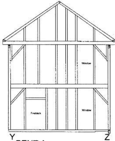
BENT A
