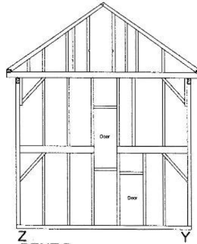
BENT B
